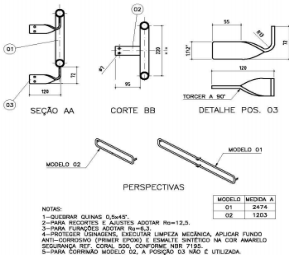
Figura 6 – Detalhes da fixação do corrimão duplo
