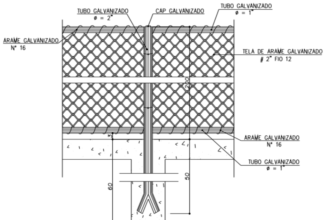
Figura 1 – Detalhamento do alambrado
