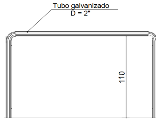
Figura 4 – Vista frontal corrimão simples fixado em piso
