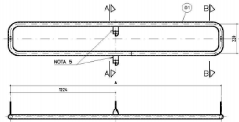
Figura 5 – Vista frontal e superior do corrimão duplo
