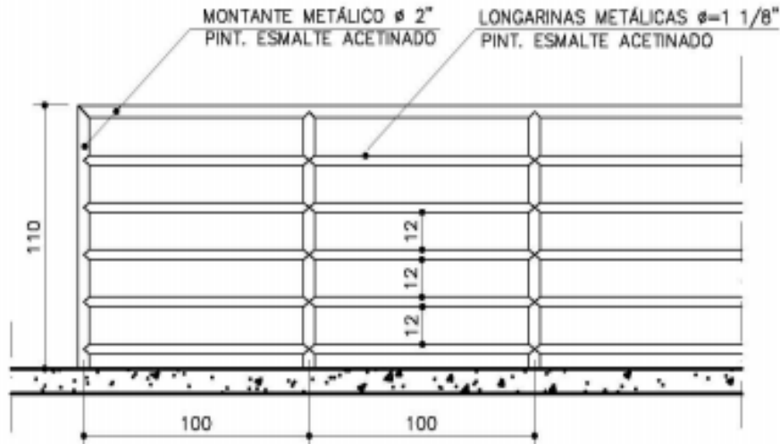
Figura 2 – Vista frontal guarda corpo de tubos horizontais
