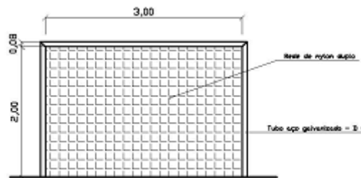
Figura 8 – Vista frontal da trave de futebol de salão
