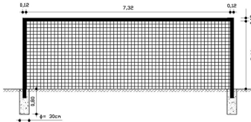
Figura 9 – Vista frontal da trave de futebol de campo
